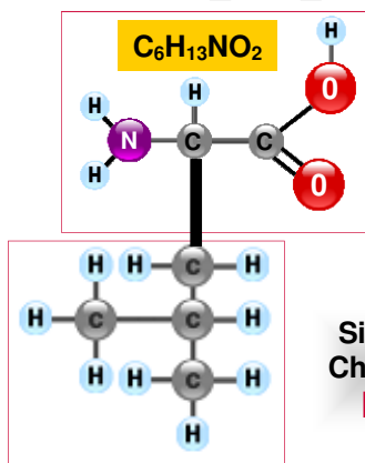
Leucine LEU_L
